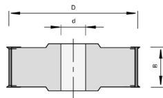
Füge-Falz Messerkopf
